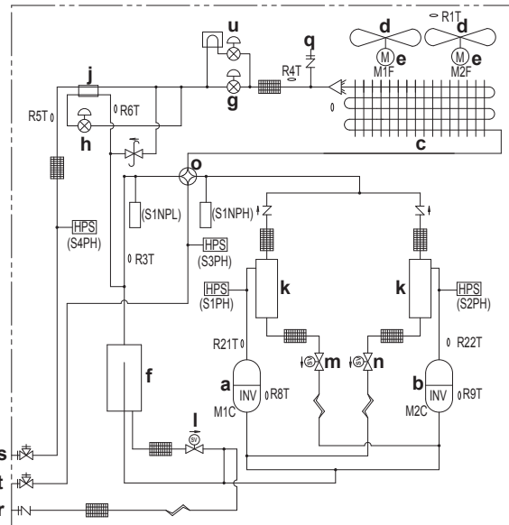
Схема трубопроводов: RXYQQ14~20
