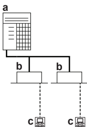
а Наружный блок VRV на основе сменного теплового насоса
