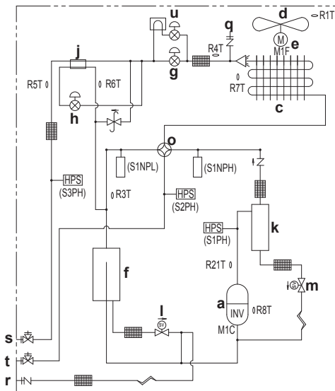
Схема трубопроводов: RXYQQ8~12
